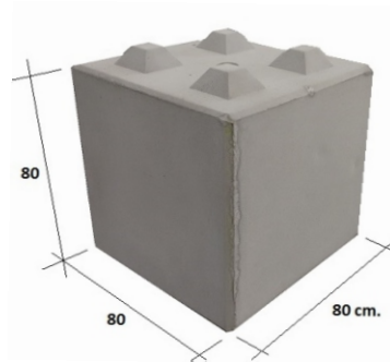
Blokazo 80 media pieza
